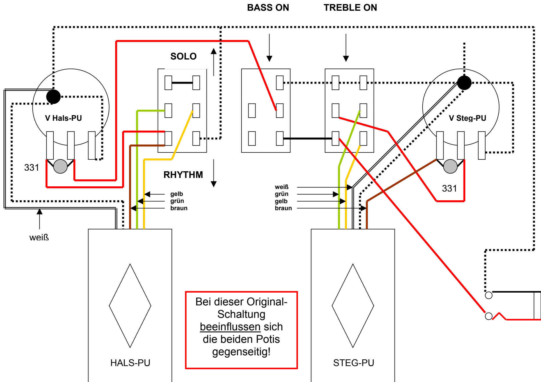
Original - Schaltplan Höfner Verythin Vintage (Bj. 2002) / 1.1
